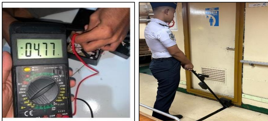
Gambar 4.22: (a) pengukuran tegangan sensor ultrasonik (b) pengetesan sensor Sumber: Dokumentasi Pribadi
