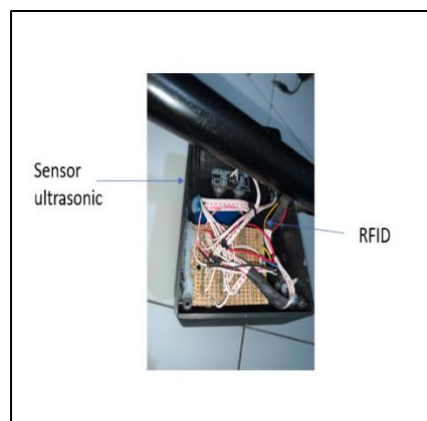
Gambar 2. Rangkaian Bawah Sumber: dokumentasi penelitian
