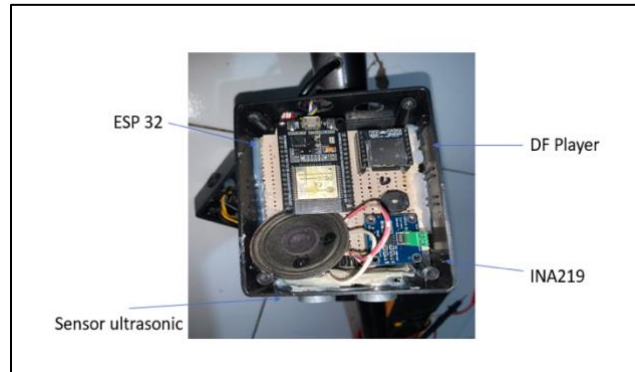
Gambar 1. Rangkaian Atas Sumber: dokumentasi penelitian
